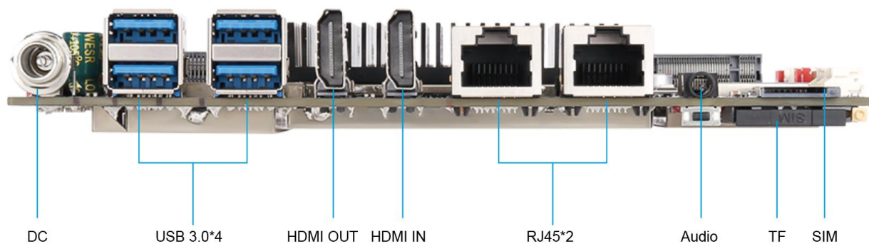
【Interface diagram】
