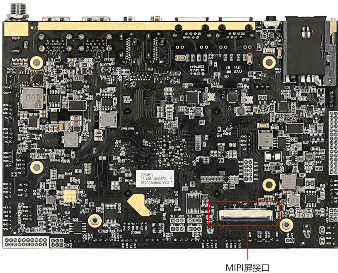
【Interface diagram】
