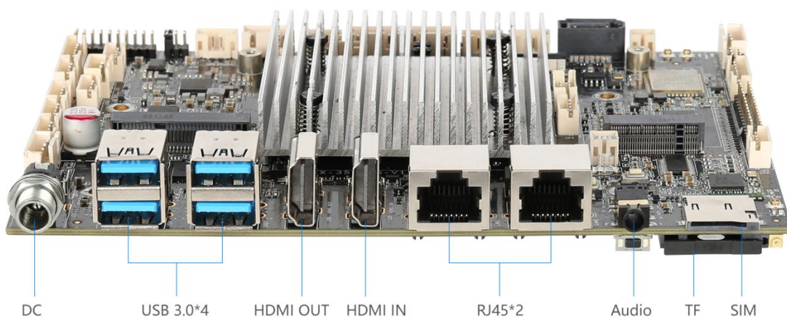
【Interface diagram】
